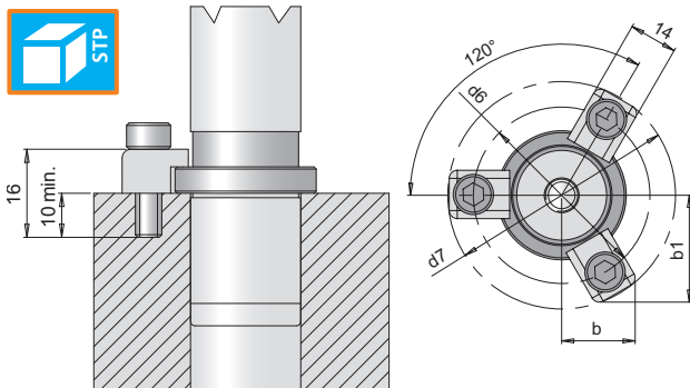
Befestigung mit Haltestück NV 3 HS 9825 Bestell-Nr.: NV 3 HS 9825.M6 bis Ø 25 mm NV 3 HS 9825.M8 ab Ø 30 mm
