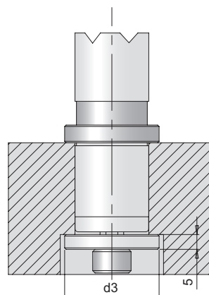
Befestigung mit Haltescheibe Bestell-Nr.: NV 3 4.d1
