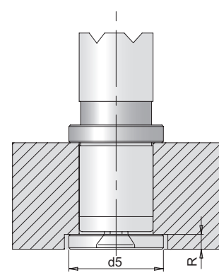
Befestigung mit Haltescheibe mit Senkkopf Bestell-Nr.: NV 3 4.S.d1
